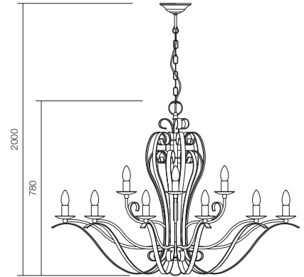
● 02-816 ● 02-817 Lampholder E14 Power 18 x max. 28W
