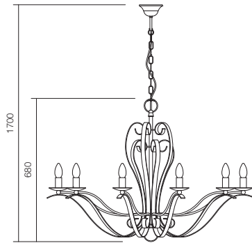
● 02-814 ● 02-815 Lampholder E14 Power 10 x max. 28W
