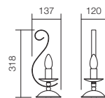
● 02-818 ● 02-819 Lampholder E14 Power 1 x max. 28W
