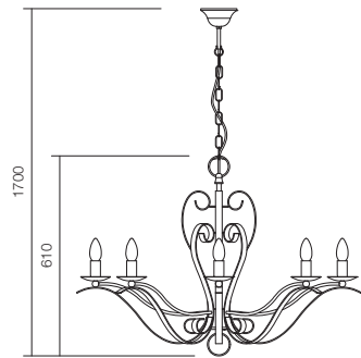
● 02-812 ● 02-813 Lampholder E14 Power 8 x max. 28W
